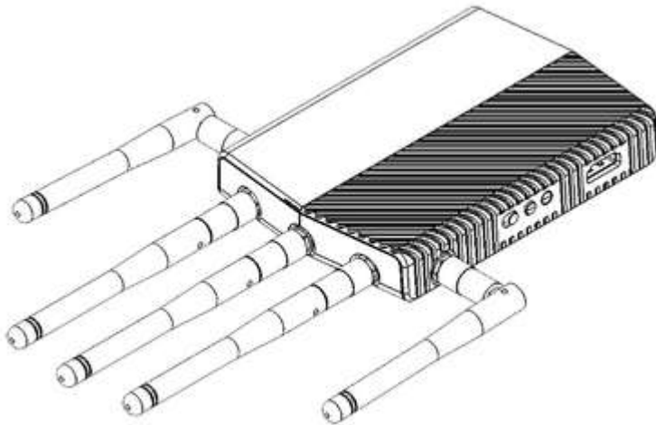
地上ユニットのアンテナの接続 - 箱 4
